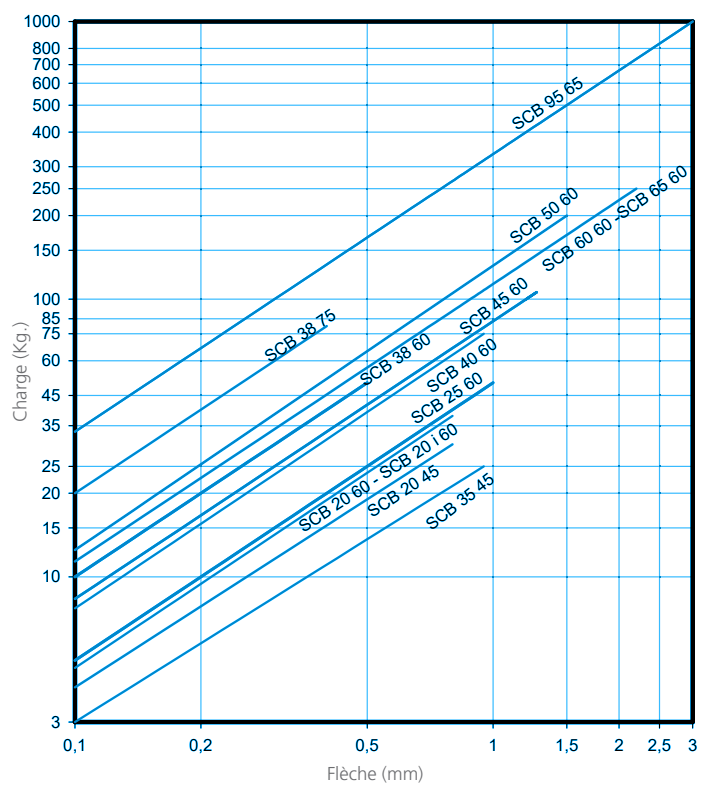
COURBE DE CHARGE-FLÈCHE AMC MECANOCAUCHO® TYPE SCB
